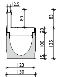
Schlitzaufsatz SW 12,5 Kl. B
