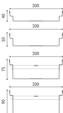
Fixe Bauhöhe
