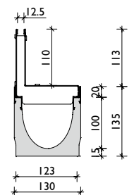
Schlitzaufsatz SW 12,5 Kl. C
