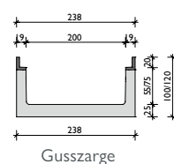
Gusszarge
