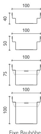
Fixe Bauhöhe
