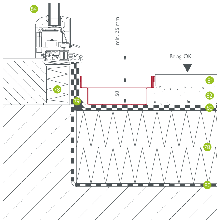
BG-FLEX FA Fassade, RB 130, Türeinbau
