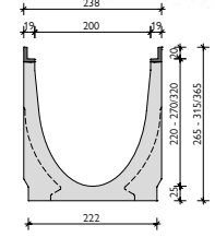
Gusszarge
