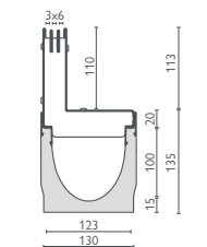
Schlitzaufsatz 3S, Heelproof SW 3x6, Kl. C
